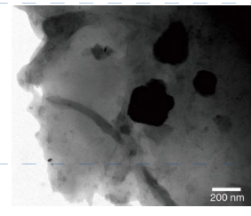
水泥-TEM
