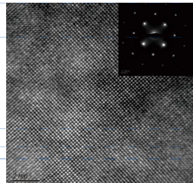
单晶硅-HRTEM
