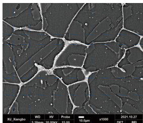
金属晶粒组织
