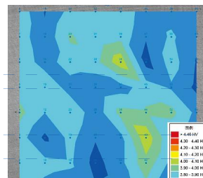
硬度分布
