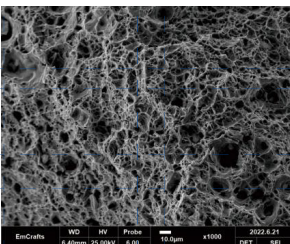
金属断面
