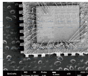
开封后的芯片
