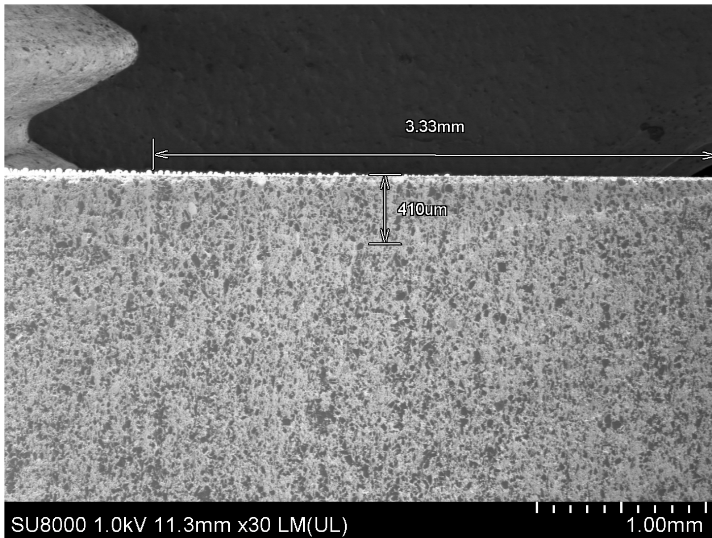
TIC3X离子束切割区域宏观图像 X30
