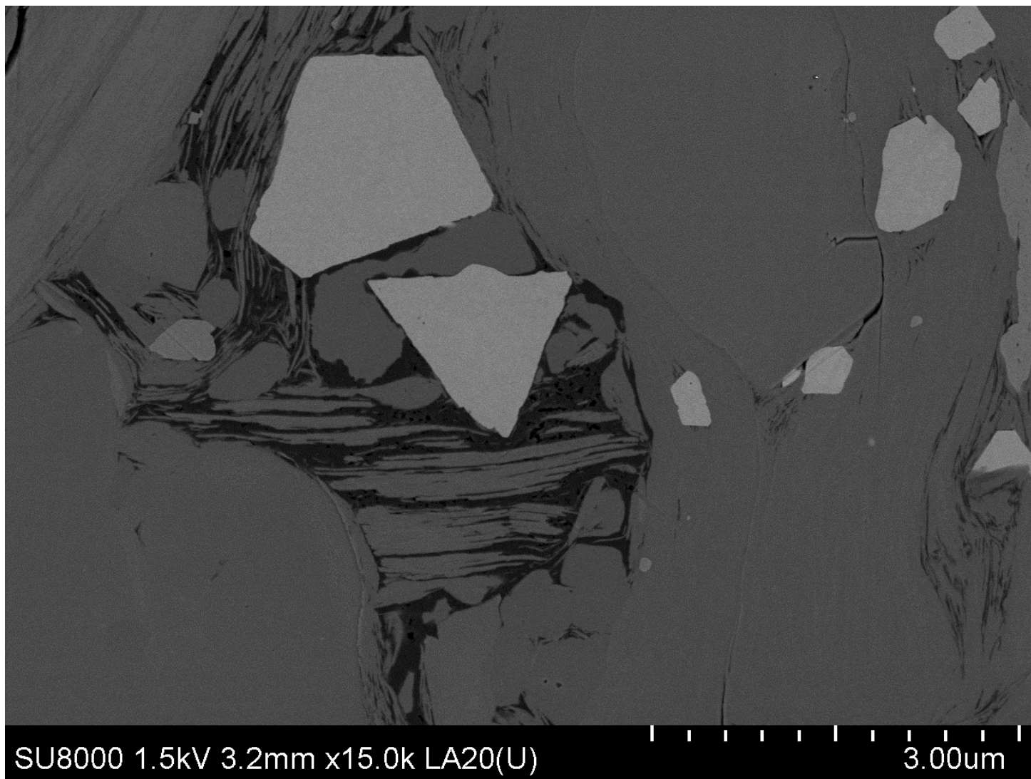
页岩气样品2: X15000
