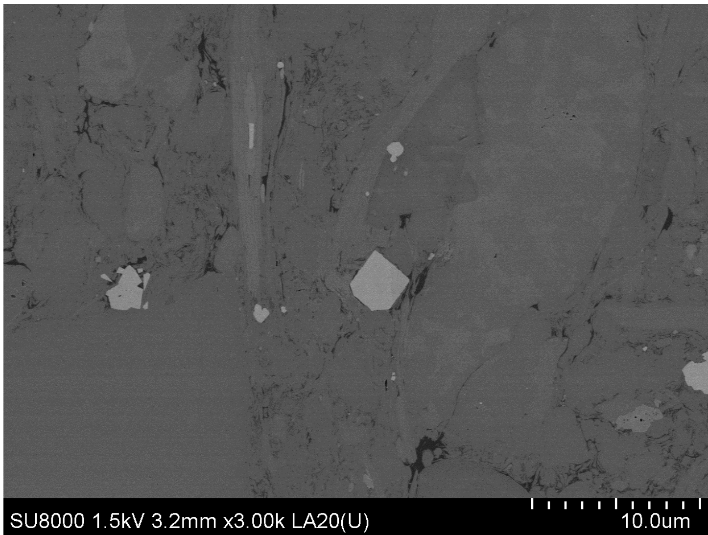
页岩气样品2： X3000
