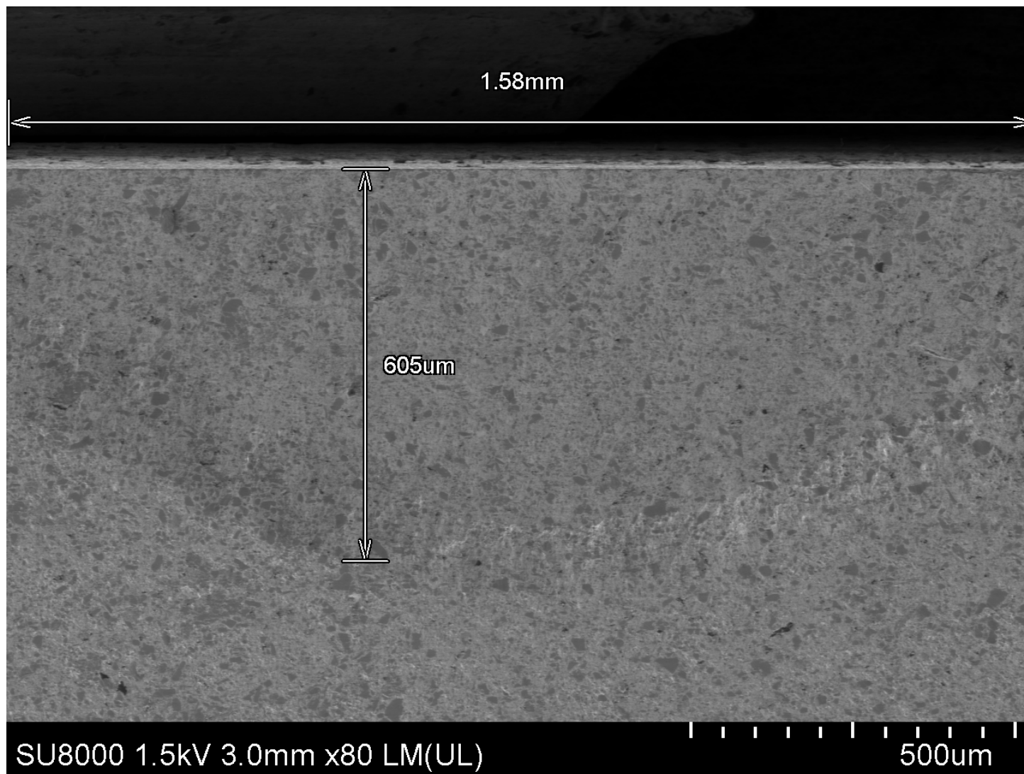
TIC3X离子束切割区域宏观图像 X80
