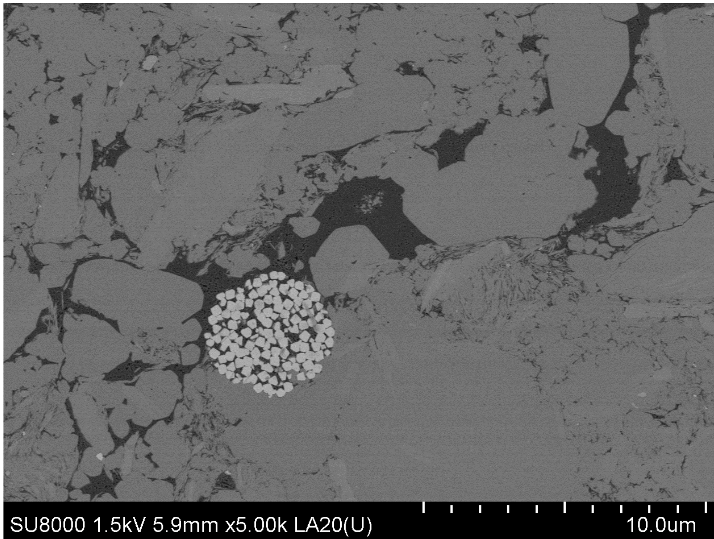
页岩气样品1： X5000
